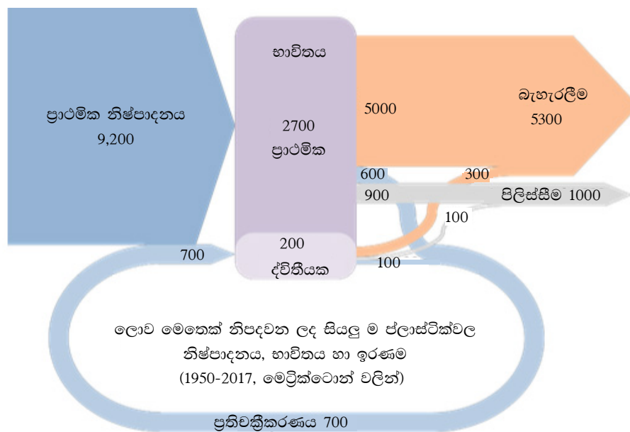
5.3.2 රූපය - 1950 සිට 2017 දක්වා නිපදවන ලද සියලු ප්ලාස්ටික්වල නිෂ්පාදනය, භාවිතය සහ ඉරණම (මෙට්‍රික් ටොන්වලින්) මූලාශ්‍රය : Geyer, 2020
